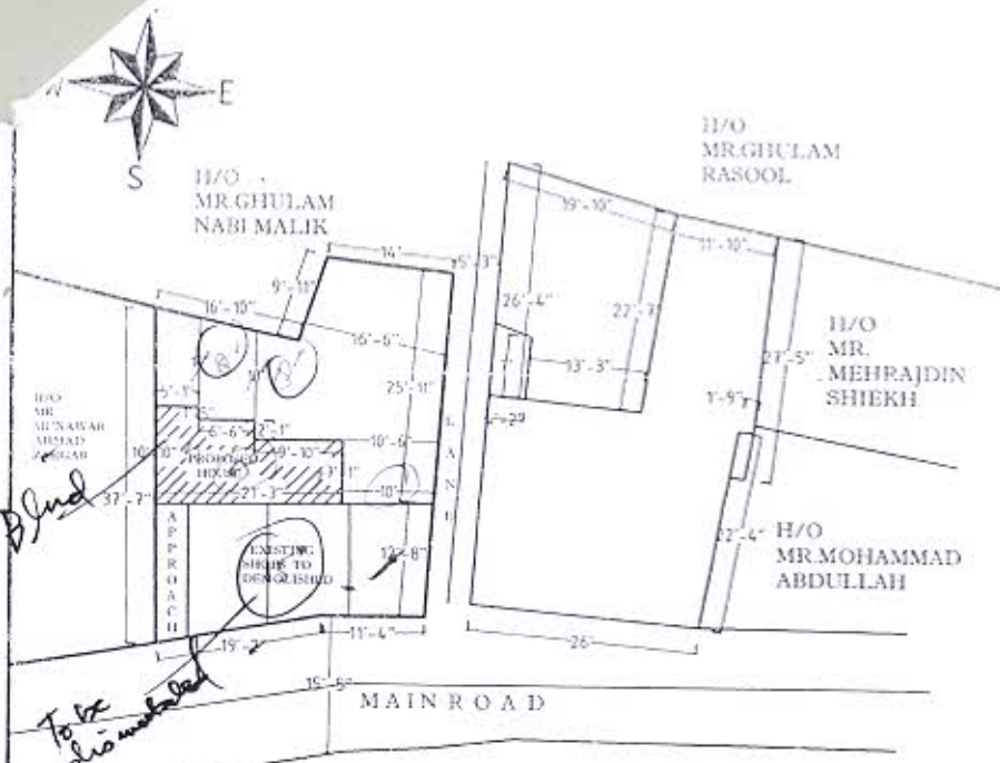
(SITE PLAN)
